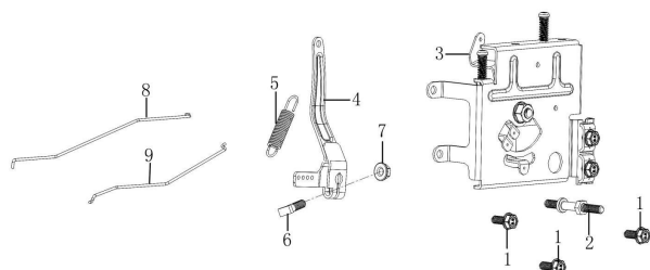
Sistema de controle
